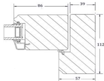
Frame Jamb & End Stile
