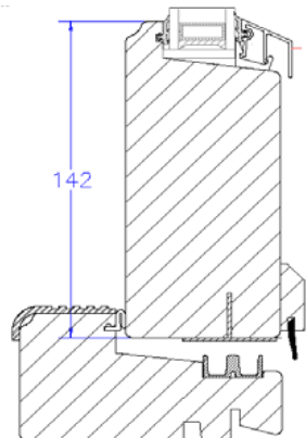
Frame Jamb & End Stile
