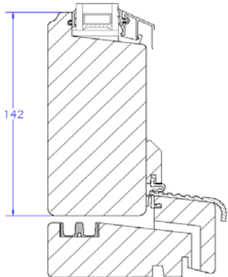
Door meeting stiles
